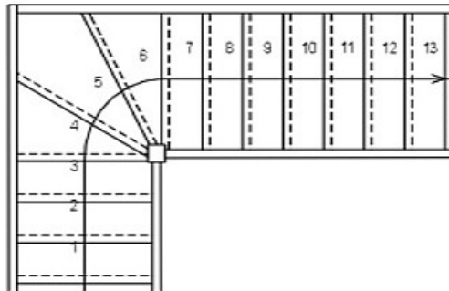
1/4 Wendelung oben nach links
