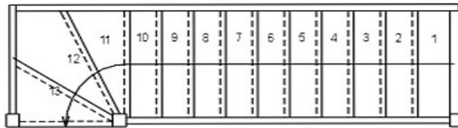
1/4 Wendelung oben nach rechts
