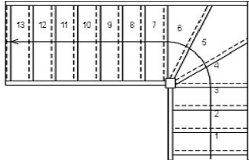
1/4 Wendelung nach rechts
